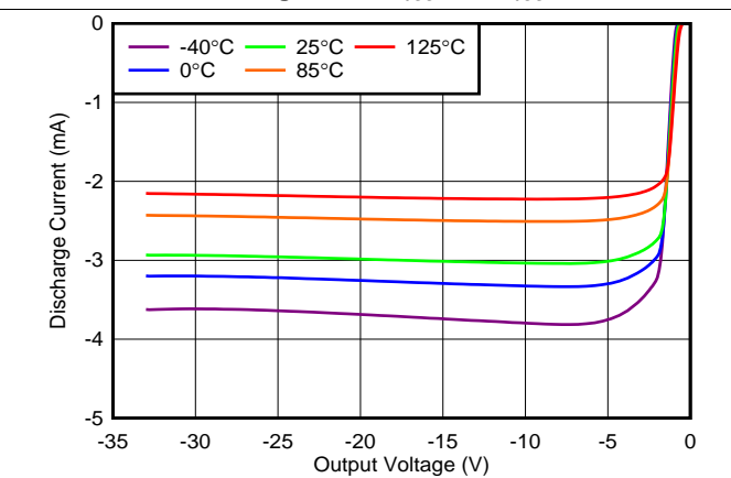
Figure 53. I_{NR/SS} vs V_{NR/SS}
